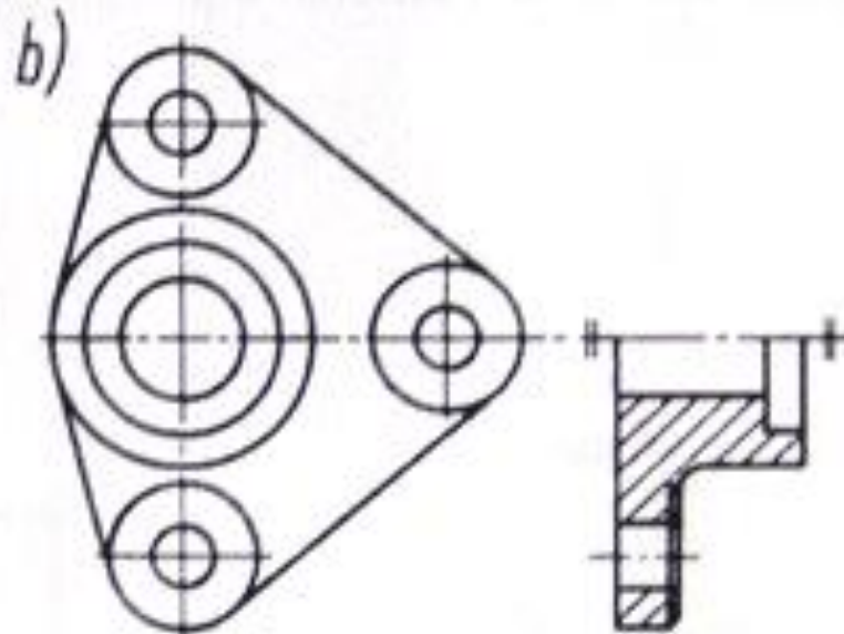
Półprzekrój
