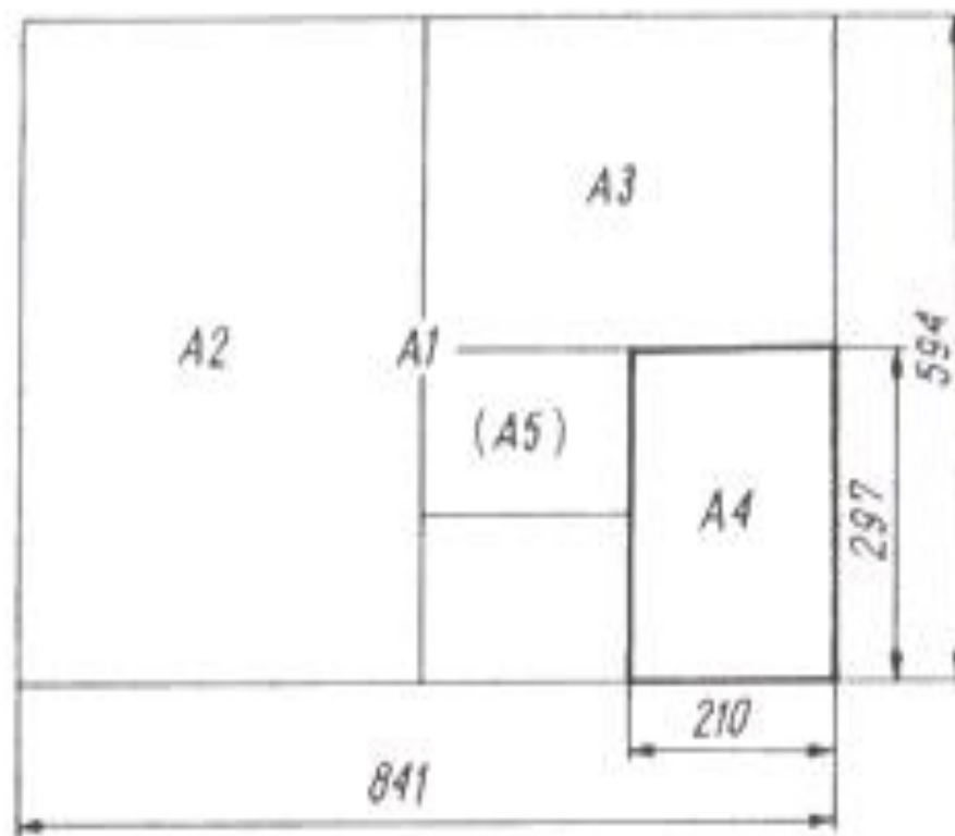
Rys. 1. Tworzenie z formatu A4 formatów podstawowych
