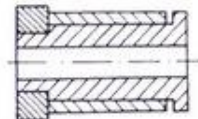
Kreskowanie płaszczyzn przekrojów stykających się elementów
