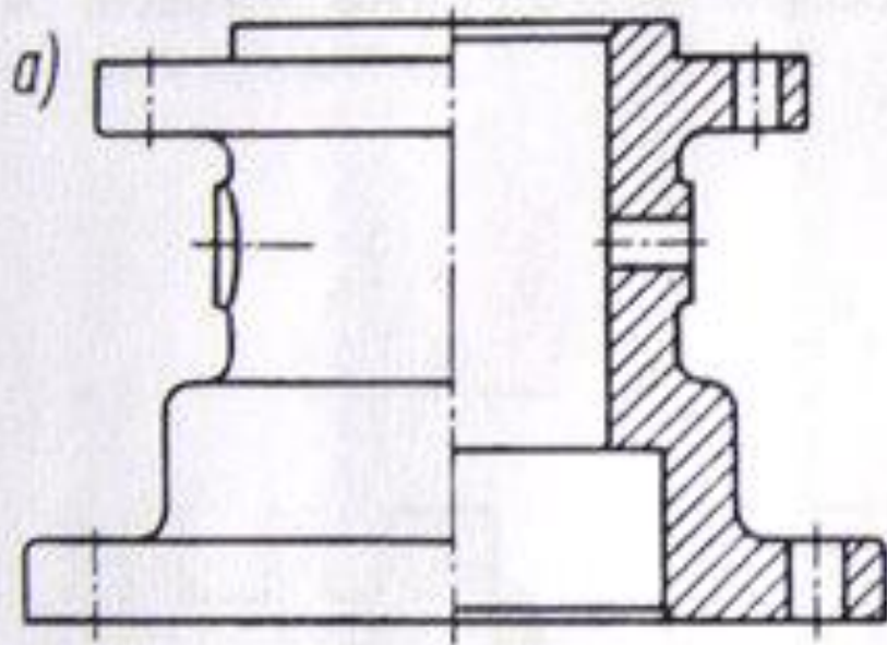
Półwidok-półprzekrój
